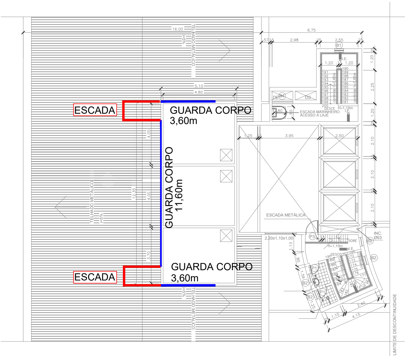
PLANTA BAIXA - POSICIONAMENTO NA COBERTURA SEM ESCALA
